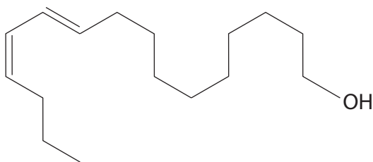
bombykol
