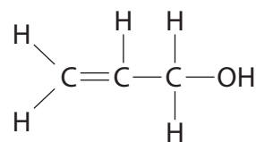
prop-2-en-1-ol
